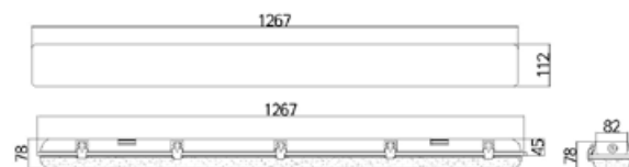
■ 슬림 방습등 Size_ W1267×D112×H78 Lamp_ LED 40W
