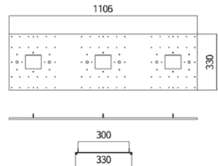
■ 크리스탈 거실 6등용 거치대 Size_ W1106×D330×H25 별도 판매
