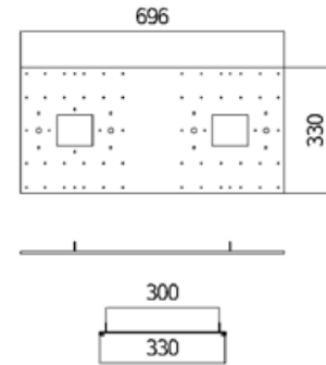
■ 크리스탈 거실 4등용 거치대 Size_ W696×D330 별도 판매
