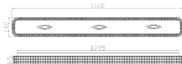
■ 크리스탈 주방등 大 Size_ W1131×D133×H85 Lamp_ LED 50W
